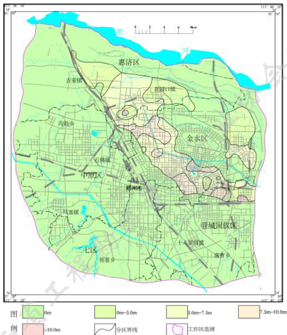
图 5-3 郑州市主城区软弱土分布及埋深图
