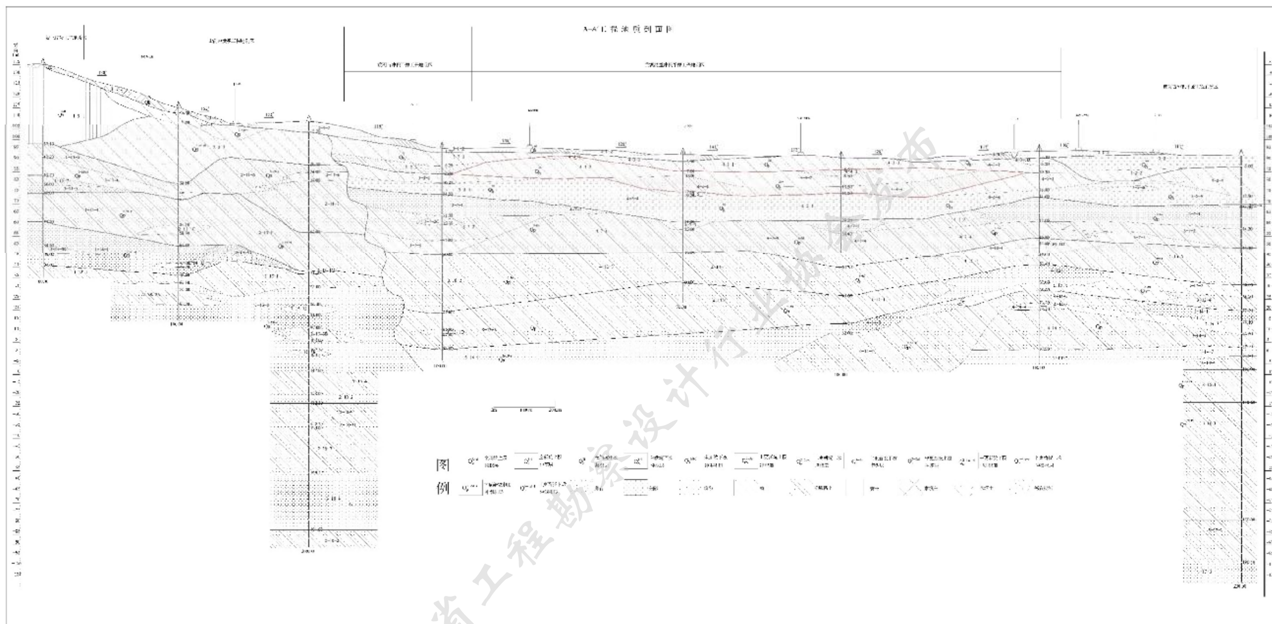
图 B.2 A-A' 工程地质剖面图
