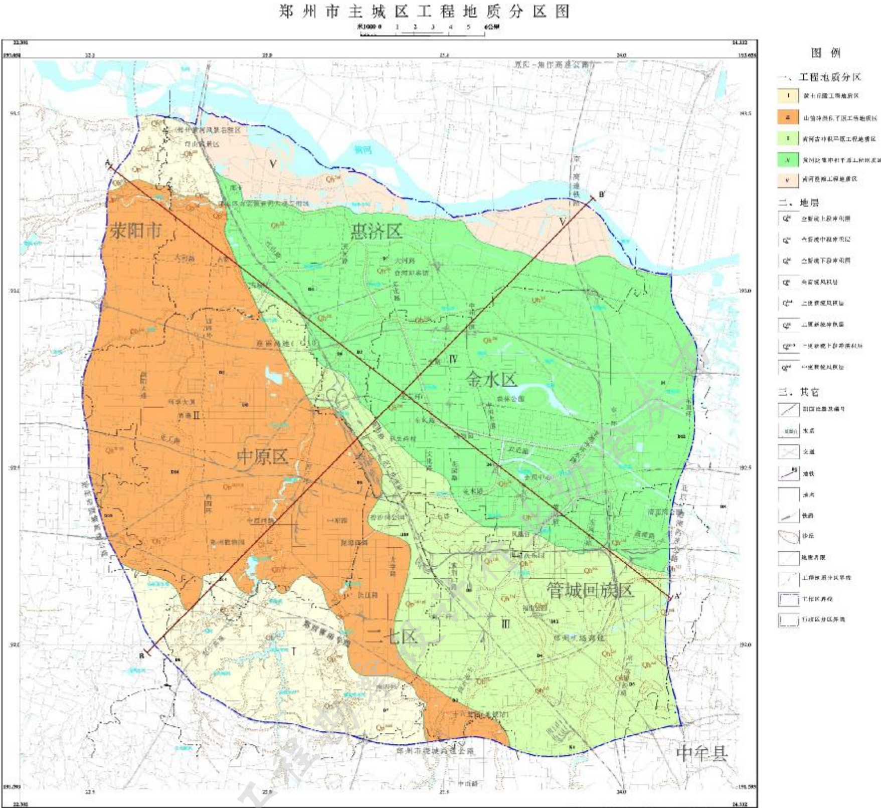
图 B.1 郑州市主城区工程地质分区图
